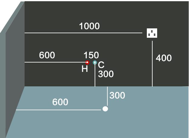
左裙水电安装图
