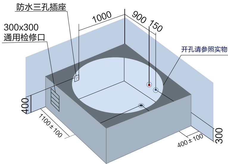
左裙水电安装图
