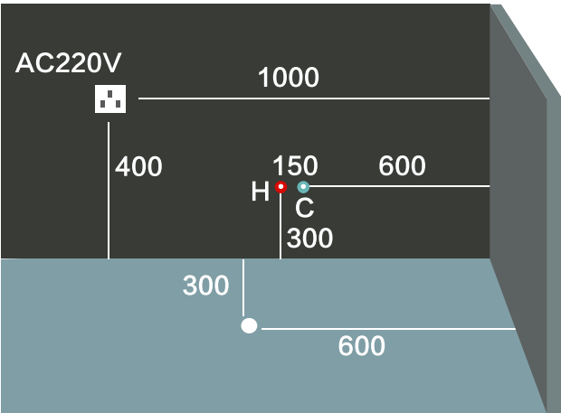
右裙水电安装图
